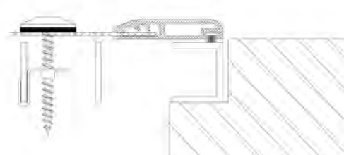
Befestigungsvariante 2 Klemmutter
