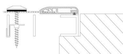
Befestigungsvariante 2 Klemmutter
