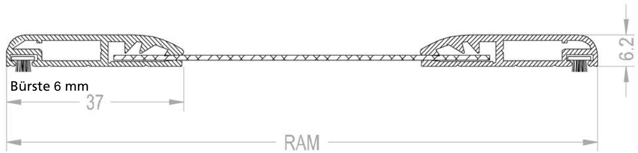
Befestigungsvariante 1 Butyl Dichtband
