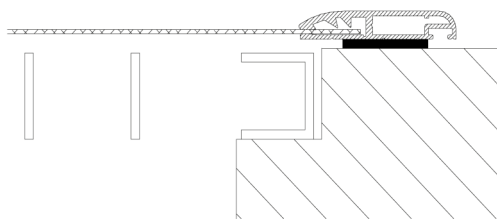
Befestigungsvariante 1 Butyl Dichtband
