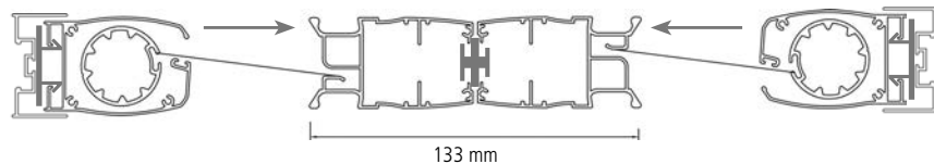
Montageprofil
