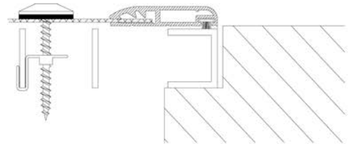
Befestigungsvariante 2 Klemmutter
