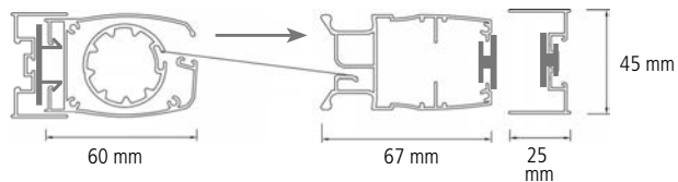
Montageprofil
