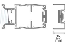
Montageprofil
