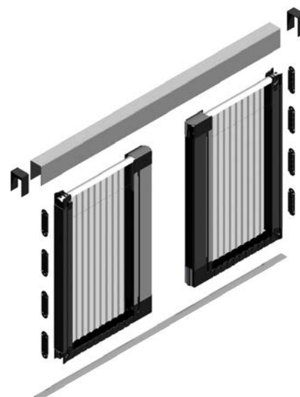
Montageprofil
