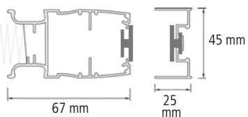
Magnetprofil
