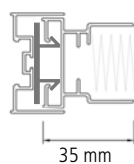
Montageprofil
